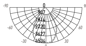
PTR 2260 60W
