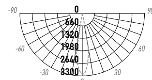
PTR 1512 12W
