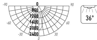
MTR16 1212 12W
