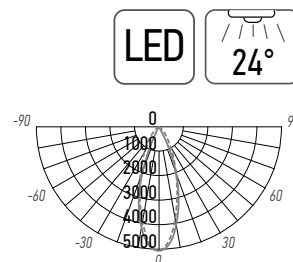
PTR 0708 8W
