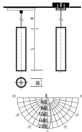
PTR 2310 10W
