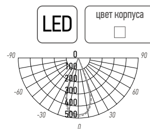
PSP-S 7W
