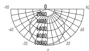
PSL 08 100W 120°
