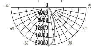
PTR 1335 35W
