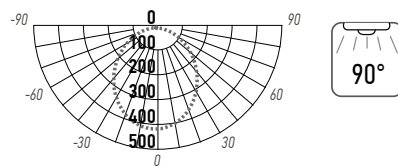
MTR16 1012 12W
