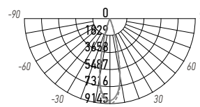
PTR 0728 28W 15°
