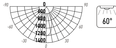
MTR16 1412 12W
