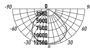
PFL-V 300W
