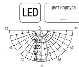
PSP-R 7W
