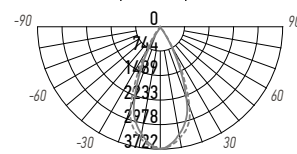
PTR 0728 28W 60°
