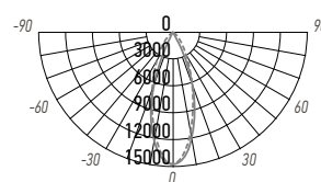
PTR 0325 25W
