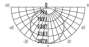
PTR 2260 60W
