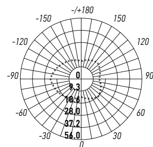
PWL-120120/0-90D 4X2W
