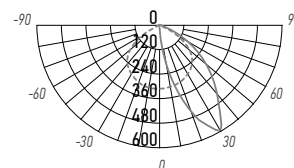
PFL-AS 50W
