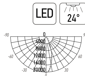
PTR 0732 32W
