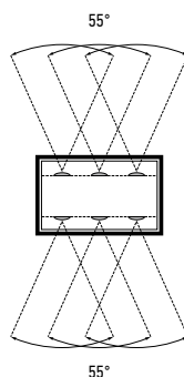
Светораспределение PWL
