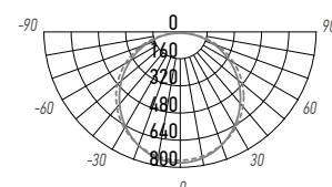
PWP-OS 36W
